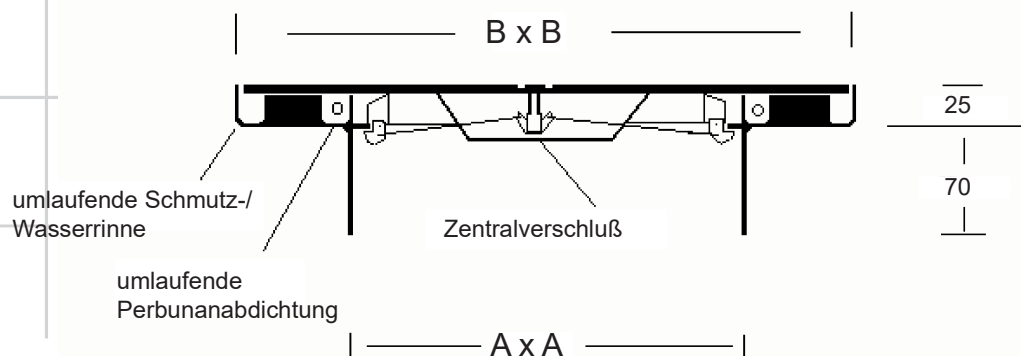
Zeichnung: befahrbare Ausführung
