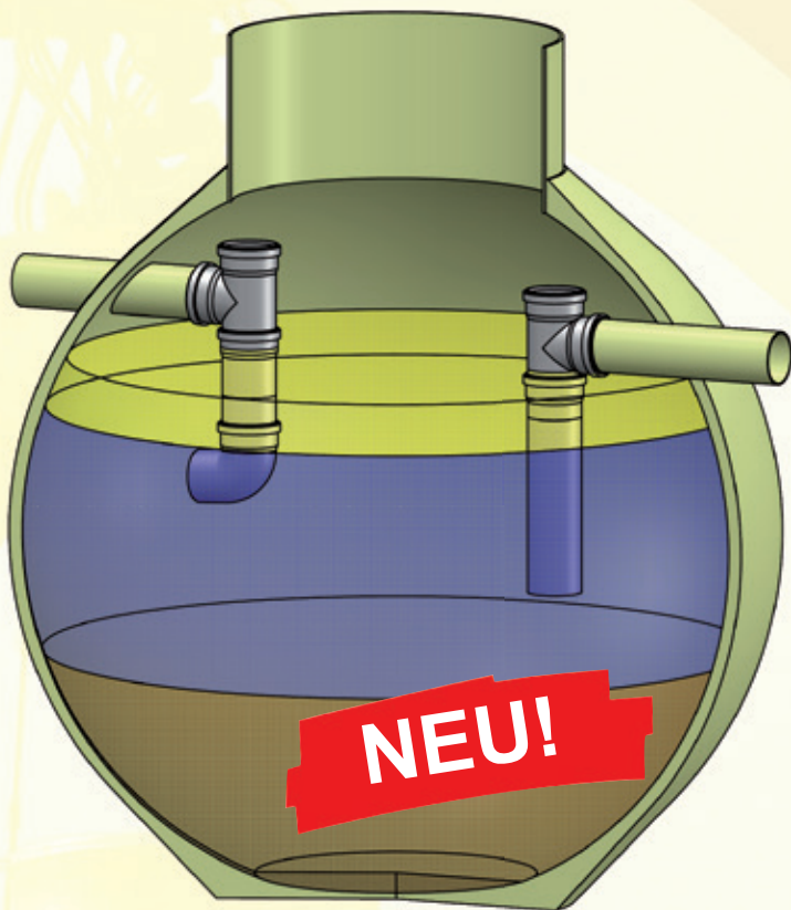
Beim Haase-Fettabscheider kommen die Vorzüge des Werkstoffs GFK besonders zur Geltung, sowohl im Tank- als auch im Schachtbereich
